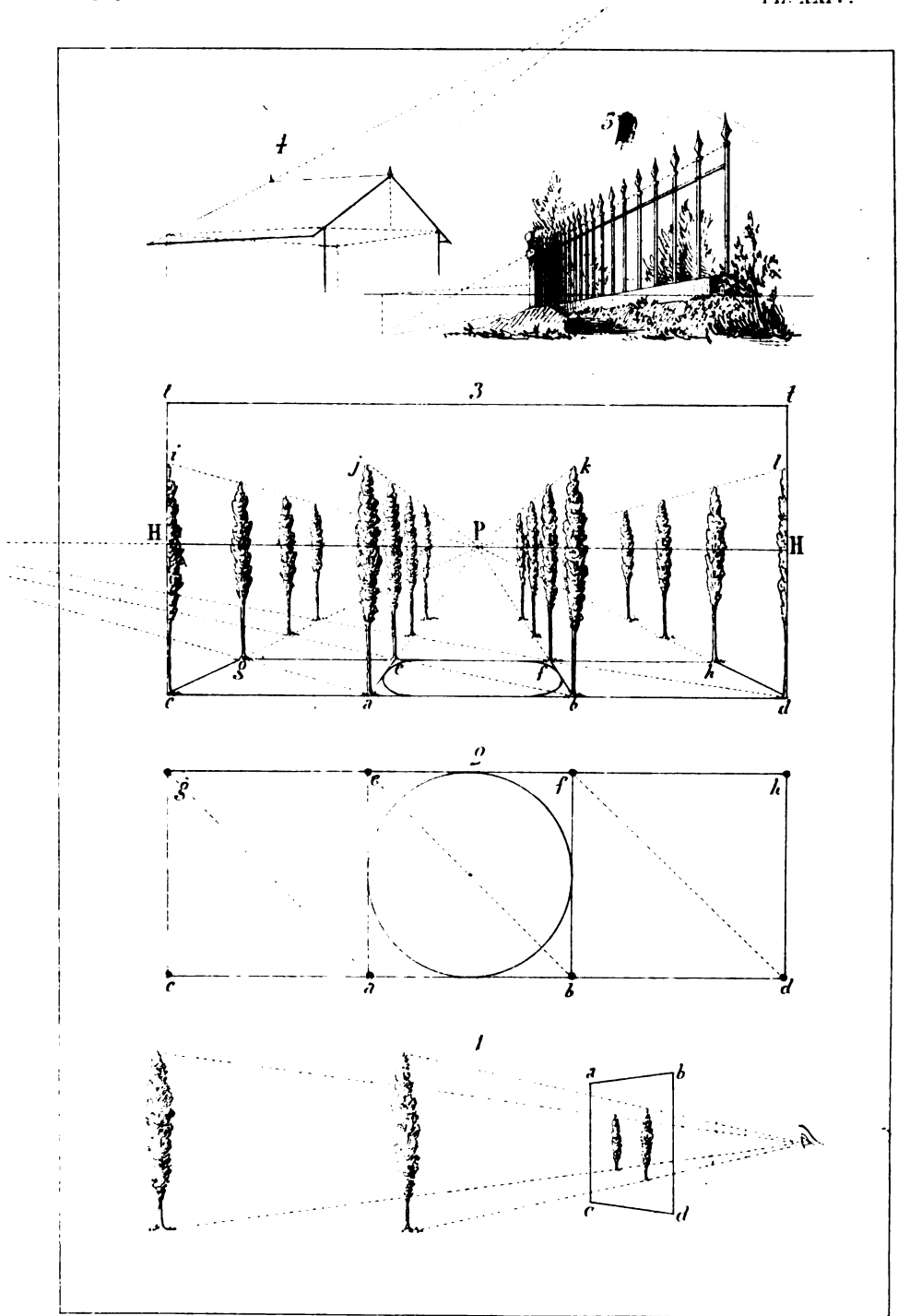
FIGURES DE PERSPECTIVE ÉLÉMENTAIRE.
